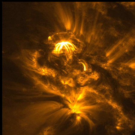
Télescope SVST, La Palma, Académie Royale des Sciences de Suède
