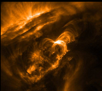
Boucles magnétiques solaires en Ultra Violet, Satellite TRACE / NASA, fausses couleurs
