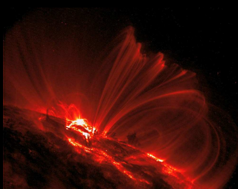
Boucles magnétiques solaires en Ultra Violet, Satellite TRACE / NASA, fausses couleurs
