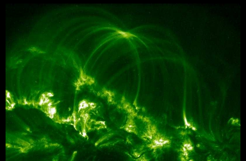
Boucles magnétiques solaires en Ultra Violet, Satellite TRACE / NASA, fausses couleurs
