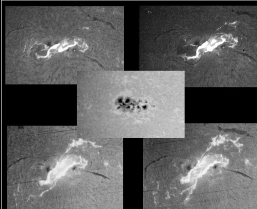
Eruption en double filet vue au spectrohéliographe de Meudon en H \alpha
