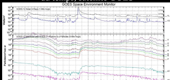
Flux de rayons X et particules en fonction du temps, satellite GOES
