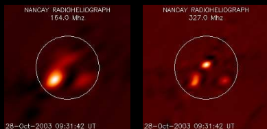
Radiohéliographe Nançay 164 et 327 MHz
