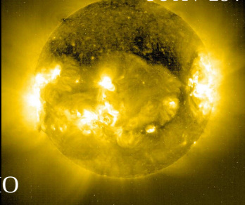
Fe XV 284
