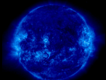
SOHO EIT
