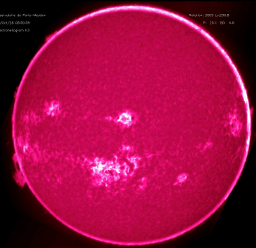
CaII K3 Meudon
