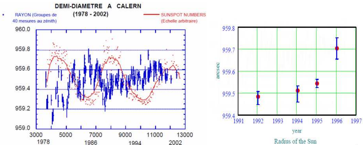
Figure 49 : Les fluctuations du rayon solaire (à gauche) pourraient être en anti corrélation avec l'activité solaire, comment le suggèrent les mesures de l'Observatoire de la Côte d'Azur au plateau de Calern. Cette hypothèse, controversée, trouve écho dans les mesures faites à partir d'un ballon stratosphérique (le Solar Disk Sextant, à droite) à 40 km d'altitude par l'équipe de l'Université de Yale (Documents G. Thuillier, LATMOS, CNRS, S. Sofia et al, Yale University).
