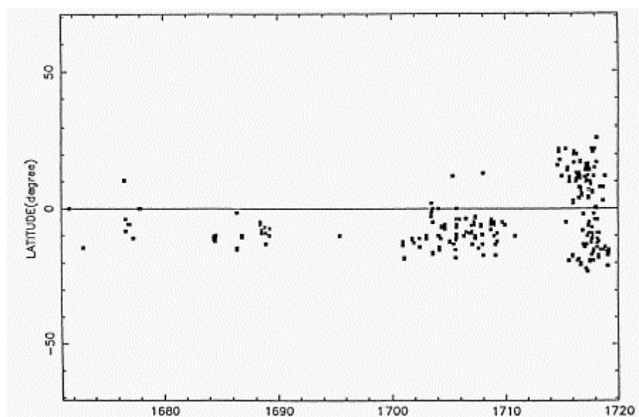
Figure 31 : Position des taches en latitude au minimum de Maunder d'après 50 ans d'observations de Picard et La Hire, interprétées par Ribes et al (1993). Noter l'anomalie de l'hémisphère Nord jusqu'en 1710 et les faibles latitudes de formation des taches autour de l'équateur. La latitude de formation ne remonte qu'à la sortie du Minimum de Maunder.
